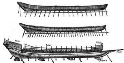
Etales de construcció d'una galera catalana
