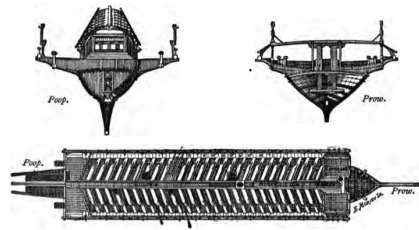
Seccions d'una galera catalana
